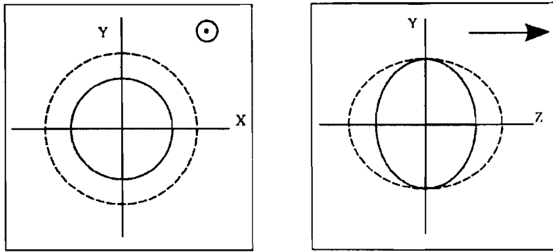
G- الحالة الأولى لاستقطاب الموجة التجاذبية
