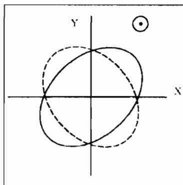
B- الحالة الثانية لاستقطاب الموجة النجاذبية الكهرمغناطيسية
