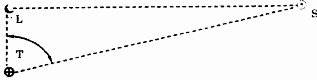
الزاوية T التي قاسها أريستارخوس بين القمر والشمس. بلغت 87 عوضاً عن 89.52 \cos 87 \approx 1/19
