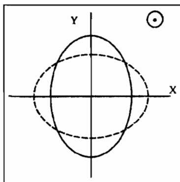
A- الحالة الأولى لاستقطاب الموجة النجاذبية الكهرمغناطيسية
