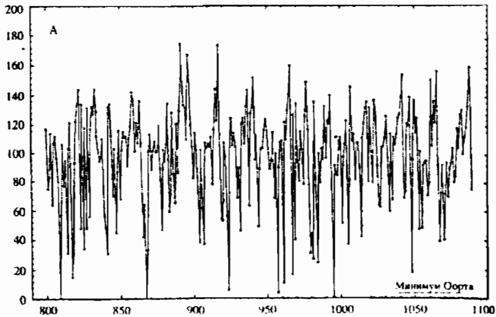
رسم بياني لتغيرات الأرقام القياسية في الزمن. الني تتصف بها الزيادة السنوية لاتساع حلقات شجرة صنوبر بين عامي ١١٠٠-١٨٠٠م
