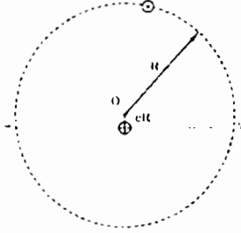
نموذج الفرض اللامتمركز (إكسنتر) عند هيبارخ فالشمس تدور حول نقطة منزاحة عن الأرض على بعد eR حيث e \approx 1/24
