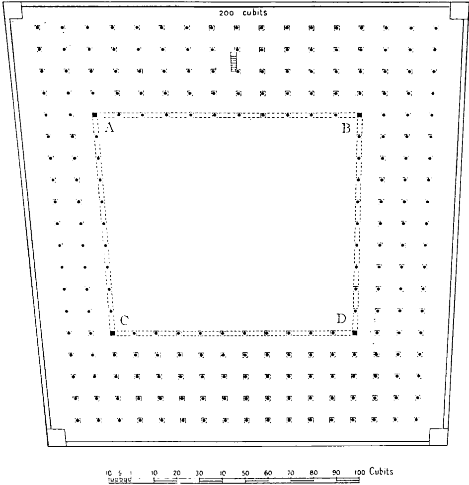
(شكل ٤) : مسقط أفقى للمسجد النبوى الشريف عقب عمارة الوليد بن عبد الملك . عن :
