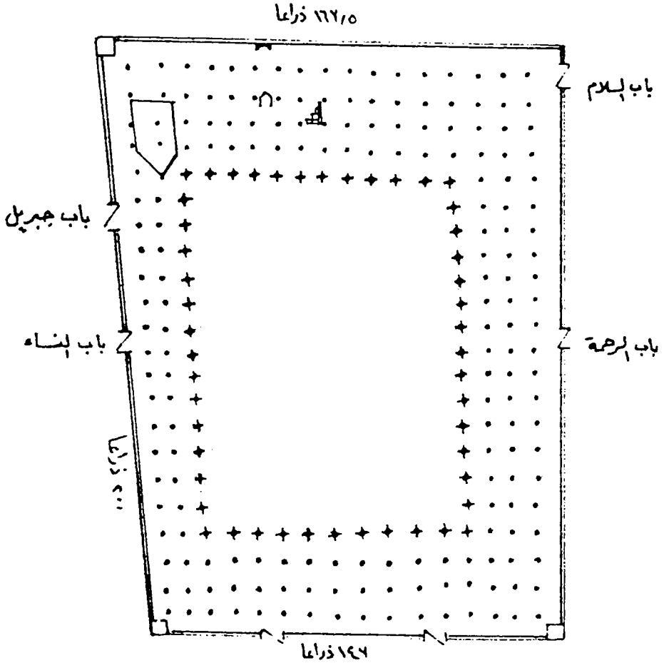
(شكل ٩) : مسقط أفقى للمسجد النبوي الشريف عقب عمارة الوليد بن عبد الملك . عن محمد هزاع الشهري.
