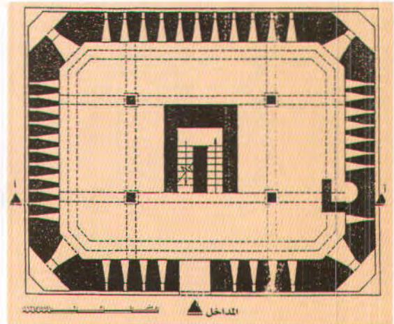
(٤٢) (عمارة القلاع والأبراج) مسقط الدور الأرضي لقلعة قباء.
