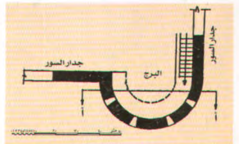
(٤٨) (عمارة القلاع والأبراج) المسقط الأفقي لبرج الكاتبية.
