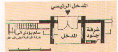
(٥٦) (عمارة القلاع والأبراج) مسقط الدور الأرضي لمدخل القلعة «الترسييس».
