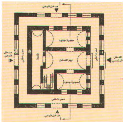
(٥١) (عمارة القلاع والأبراج) المسقط الأفقي للدور الأرضي لقلعة عروة.
