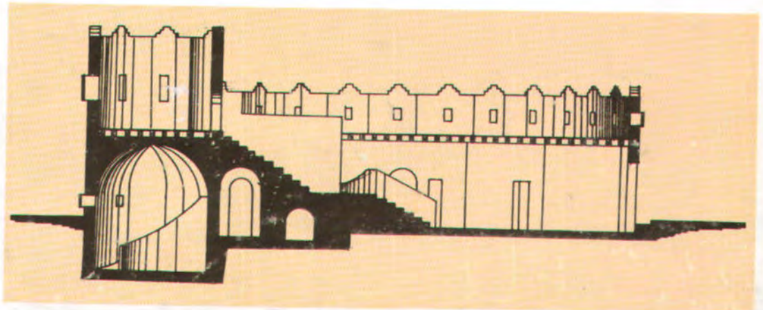
(٦١) (عمارة القلاع والأبراج) القطاع أ. الهيكل لقلعة أحد.
