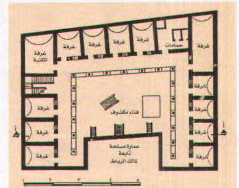
(٨٦) (الأربطة) مسقط الدور الأول والثاني لرباط مظهر الفاروقي.
