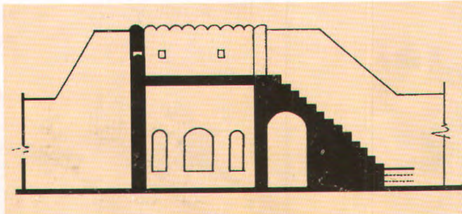
(٥٧) (عمارة القلاع والأبراج) القطاع أ-أ لمبنى مدخل القلعة «الترسييس».
