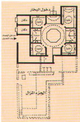
(١٠١) (الحمامات) صورة مصغرة لمسقط حمام العنبرية بعد إجراء التعديلات وهدم مدخل الحمام الرئيسي.
