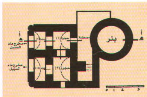
(١٠٩) (الأسبلة) المسقط الأفقي لسبيل العنبرية.
