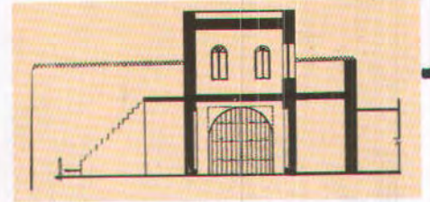
(٥٤) (عمارة القلاع والأبراج) القطاع أ-أ في برج سور الترسييس.
