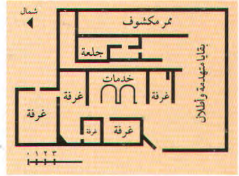
(١٦) (التنمية العمرانية) المسقط الأفقي لقصر سعيد بن العاص حسب ما يتضح من بقايا وأطلال القصر.
