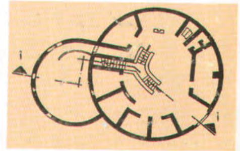
(٥٩) (عمارة القلاع والأبراج) المسقط الأفقي لقلعة أحد.
