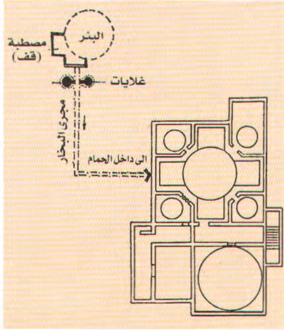
(٩٩) (الحمامات) مسقط أفقي مصغر لحمام طيبة يبين علاقة الحمام بالبئر المخصص لتزويد الحمام بالمياه ومواقع مكائن التسخين.
