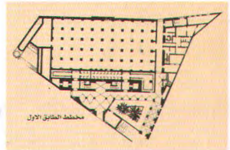
(٥) (توسعة وعمارة مسجد القبلتين) المسقط الأفقي للمستوى الأول لمسجد القبلتين في عمارته الأخيرة في عهد خادم الحرمين الشريفين (٢).
