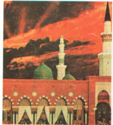
(٣٣) (المسجد النبوي) صورة للمسجد النبوي الشريف وتظهر المئذنة الرئيسية بجوار القبة الشريفة حيث تحتل الركن الجنوبي الشرقي من المسجد وهي كما بناها السلطان قايتباي، كما يظهر جزء من مئذنة باب السلام والتي أعاد بناء جزئها العلوي السلطان عبد المجيد (٥) .
