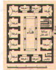
(٨٠) (المدارس) المسقط الأفقي للدور الأرضي لمدرسة حسين أغا.
