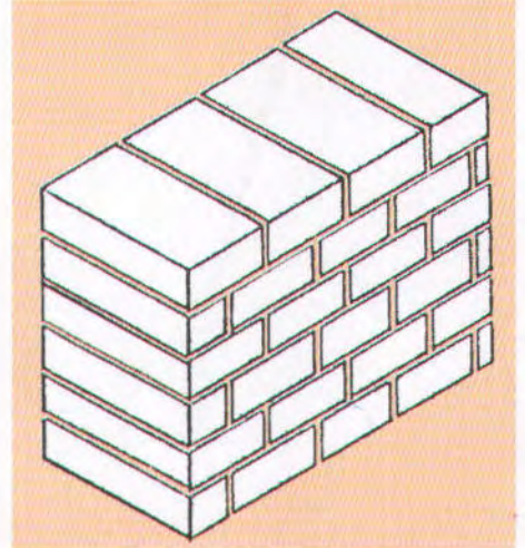
(١٧) (المسجد النبوي) نموذج البناء بالسميط «لينة على لينة» . النموذج الأول الذي استخدم في بناء المسجد النبوي الشريف وهو البناء بالسميط أي لينة على لينة .
