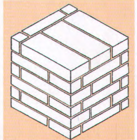
(١٨) (المسجد النبوي) نموذج البناء بالسعيدة «لينة ونصف» . النموذج الثاني الذي استخدم في بناء المسجد النبوي الشريف وبالسعيدة وهي لينة ونصف .
