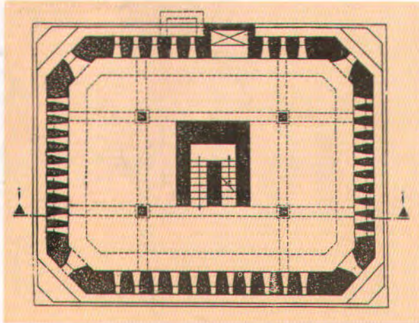
(٤٤) (عمارة القلاع والأبراج) مسقط الدور الأول لقلعة قباء.
