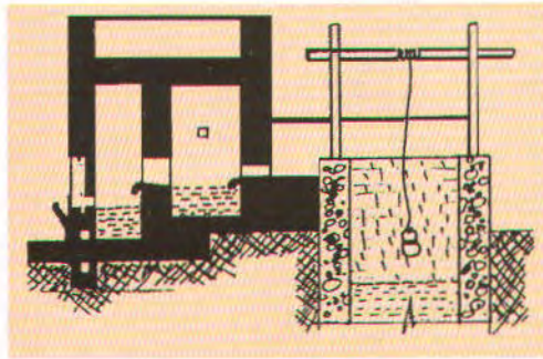
(١٠٧) (الأسبلة) القطاع أ-أ في سبيل العنبرية.
