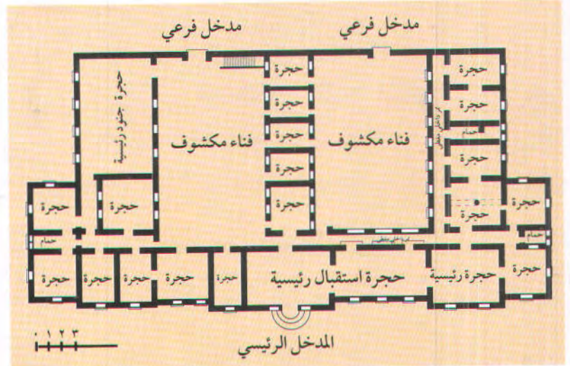
(٥٢) (عمارة القلاع والأبراج) المسقط الأفقي لمبنى الاتصالات الرئيسي «الترسييس».
