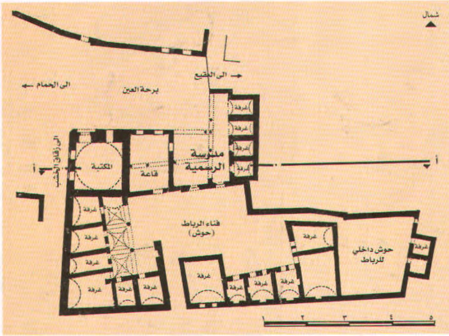
(٧٢) (المدارس) المسقط الأفقي لمدرسة ومكتبة ورباط الرستمية.
