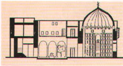
(١١٨) (المكتبات) القطاع أ. في مكتبة عارف حكمت.
