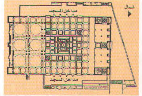
(٥) (مسجد قباء) المسقط الأفقي لمسجد قباء بعد عمارته الأخيرة في عهد خادم الحرمين الشريفين (٢) .
