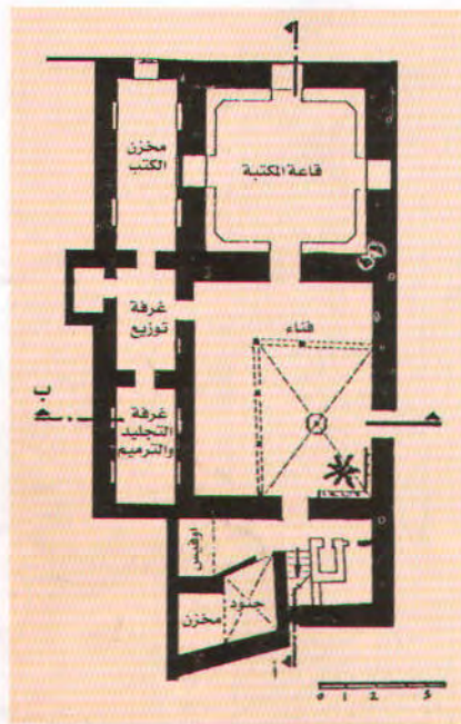
(١١٩) (المكتبات) مسقط الدور الأرضي لمكتبة عارف حكمت.
