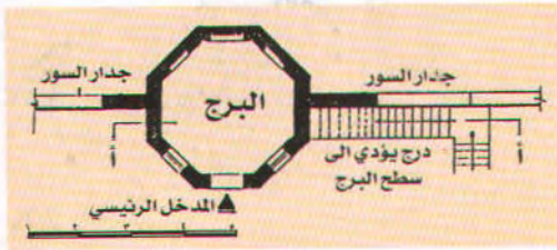
(٥٣) (عمارة القلاع والأبراج) مسقط أفقي لأحد أبراج سور الترسييس.
