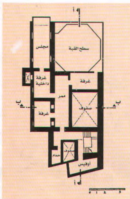
(١٢١) (المكتبات) المسقط الأفقي للدور الأول لمكتبة عارف حكمت.
