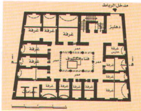
(٩٢) (الأريطة) مسقط الدور الأرضي لرباط الحيادرة.
