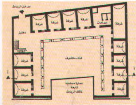
(٨٤) (الأربطة) مسقط الدور الأرضي لرباط مظهر الفاروقي.
