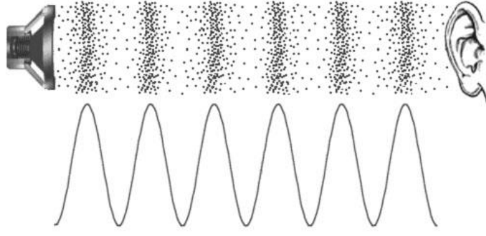
الشكل رقم (1) يبين التضاضعات والتخلخلات في حركة جزيئات الهواء، فكل تضاضع يقابله
