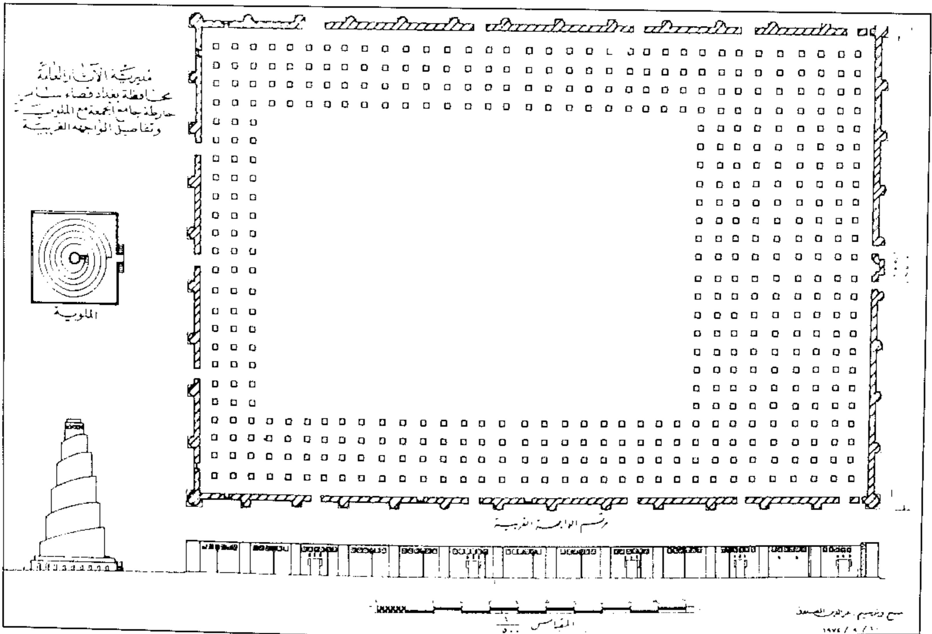
مخطط المسجد الجامع مع الملوية وتفاصيل الواجهة الغربية
